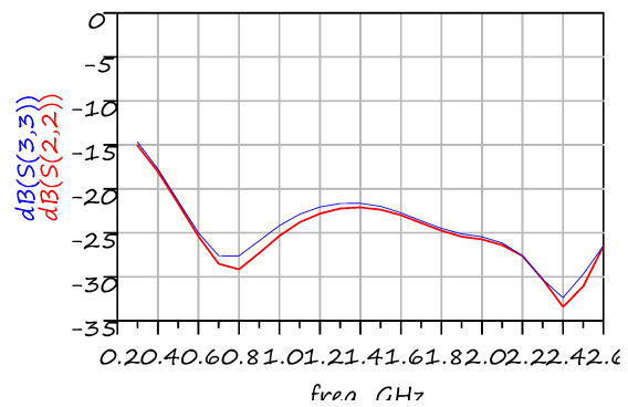
输出回波 vs 频率
