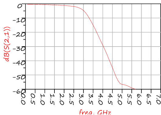
带外抑制 vs 频率
