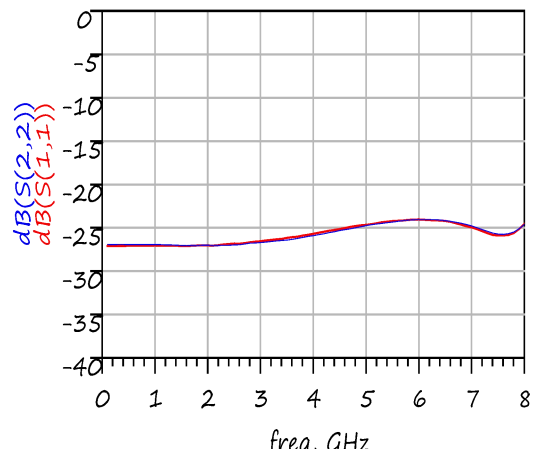
输入输出回波 vs 频率
