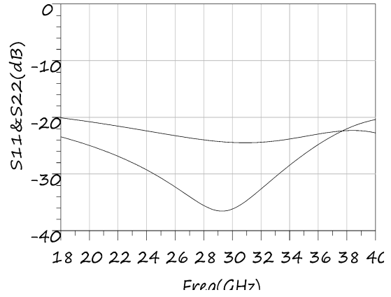
输入输出回波 vs 频率
