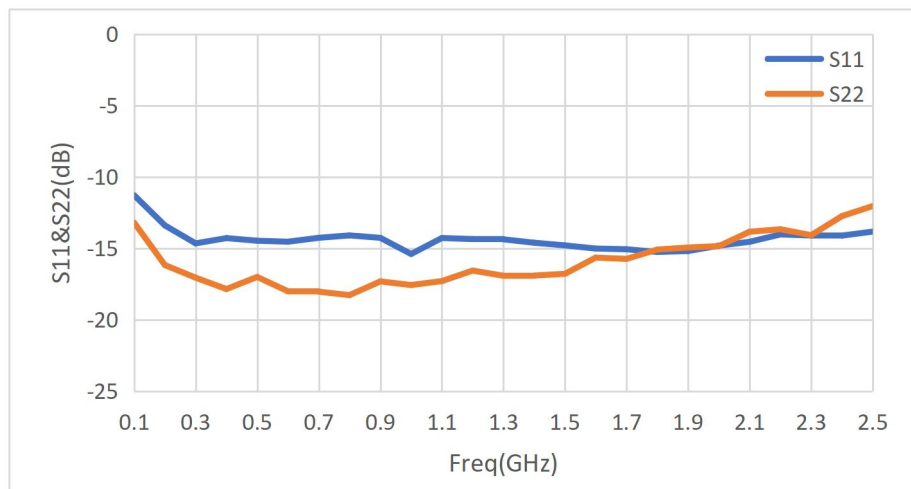
输入输出回波 vs 频率
