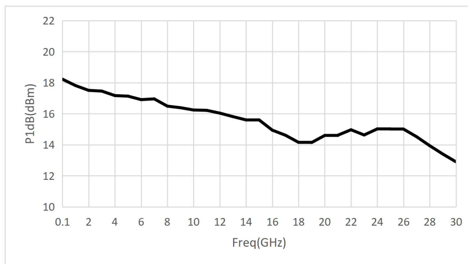
1dB 压缩输出功率 vs 频率
