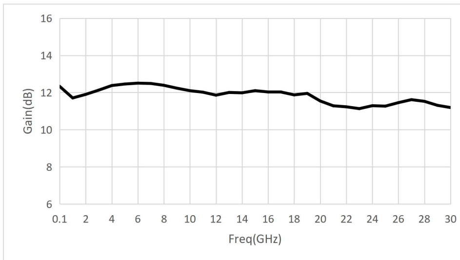
增益 vs 频率
