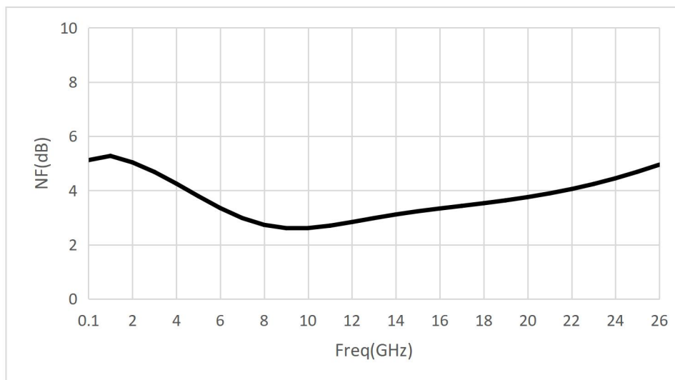
噪声系数 vs 频率
