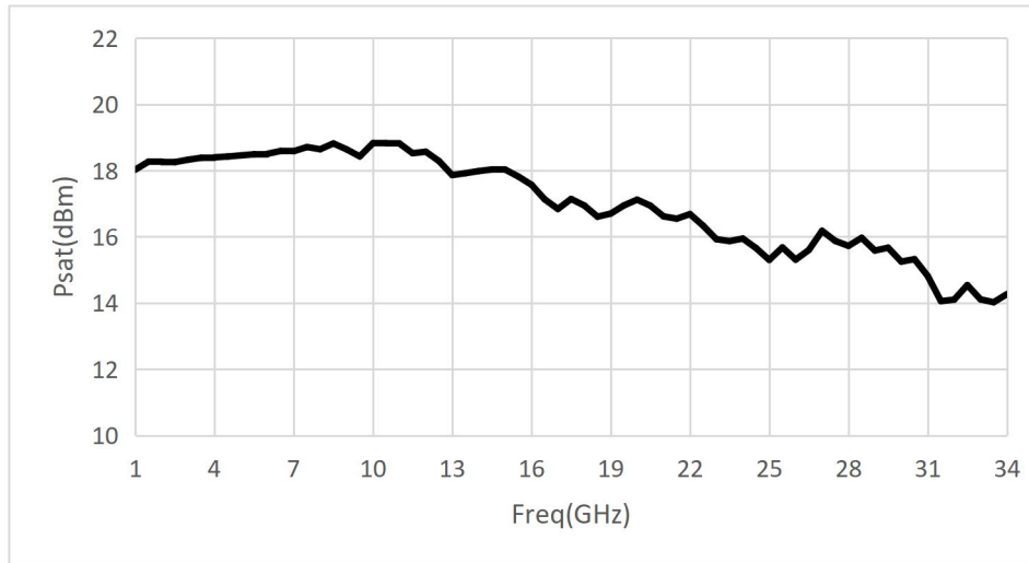
饱和输出功率 vs 频率
